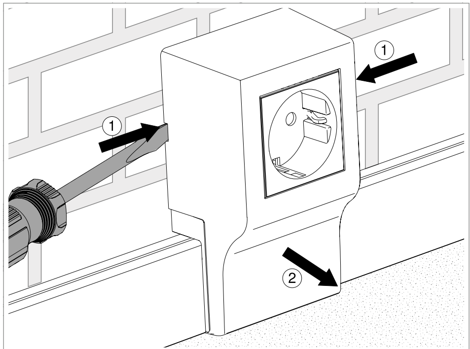
Fig. 32: Geräteträger demontieren
